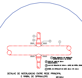
DETALHE DE INTERLIGAÇÃO ENTRE REDE PRINCIPAL E RAMAL DE SPRINKLERS
