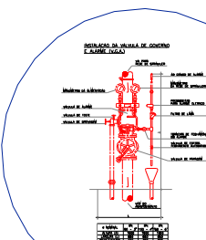
INSTALAÇÃO DA VÁLVULA DE GOVERNO
