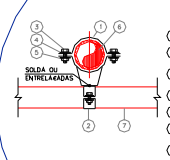
SUPOORTE EM ESTRUTURA METÁLICA (SUPOORTE TIPO S6)
