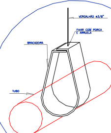
DETALHE DA BRACADEIRA
